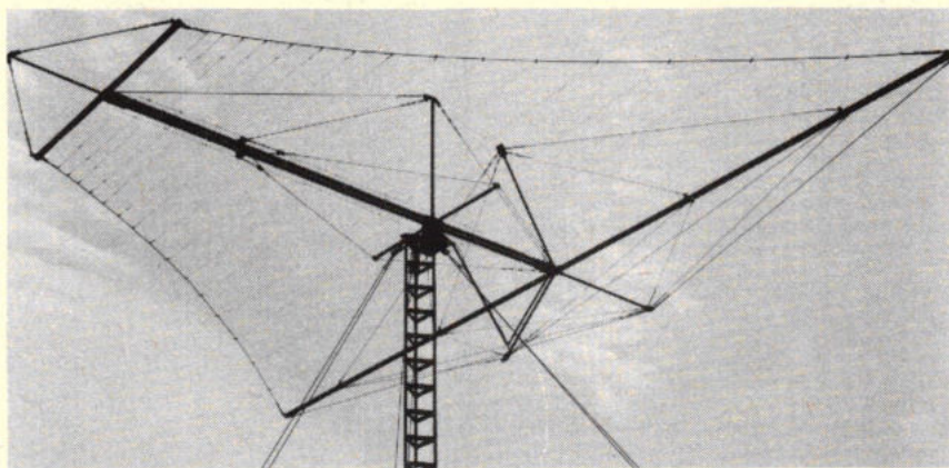
Rohde & Schwarz ontwikkelde een draaibare, logarithmisch-periodische dipoolantenne met een heel speciale vormgeving. Deze antenne van de typeserie AK 7... en AK 8... is geschikt voor het frequentiebereik van 5 tot 30 MHz ten behoeve van communicatieverkeer over middelgrote en grote afstanden. (foto: Rohde & Schwarz)
